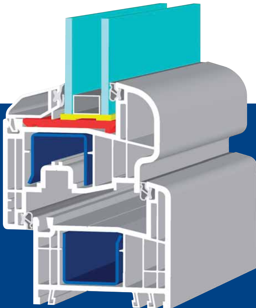
profilé à 6 chambres
