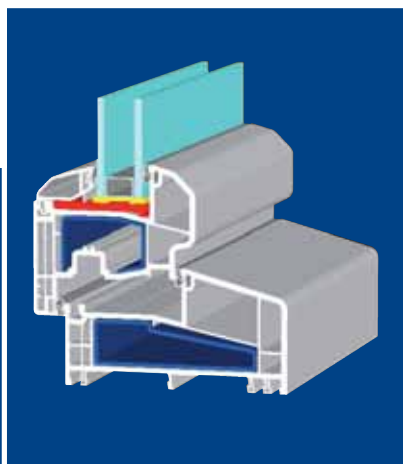
fenêtre-bloc (style hollandais)
