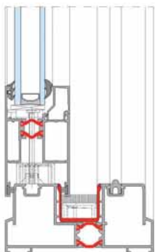
Section d'une porte coulissante
